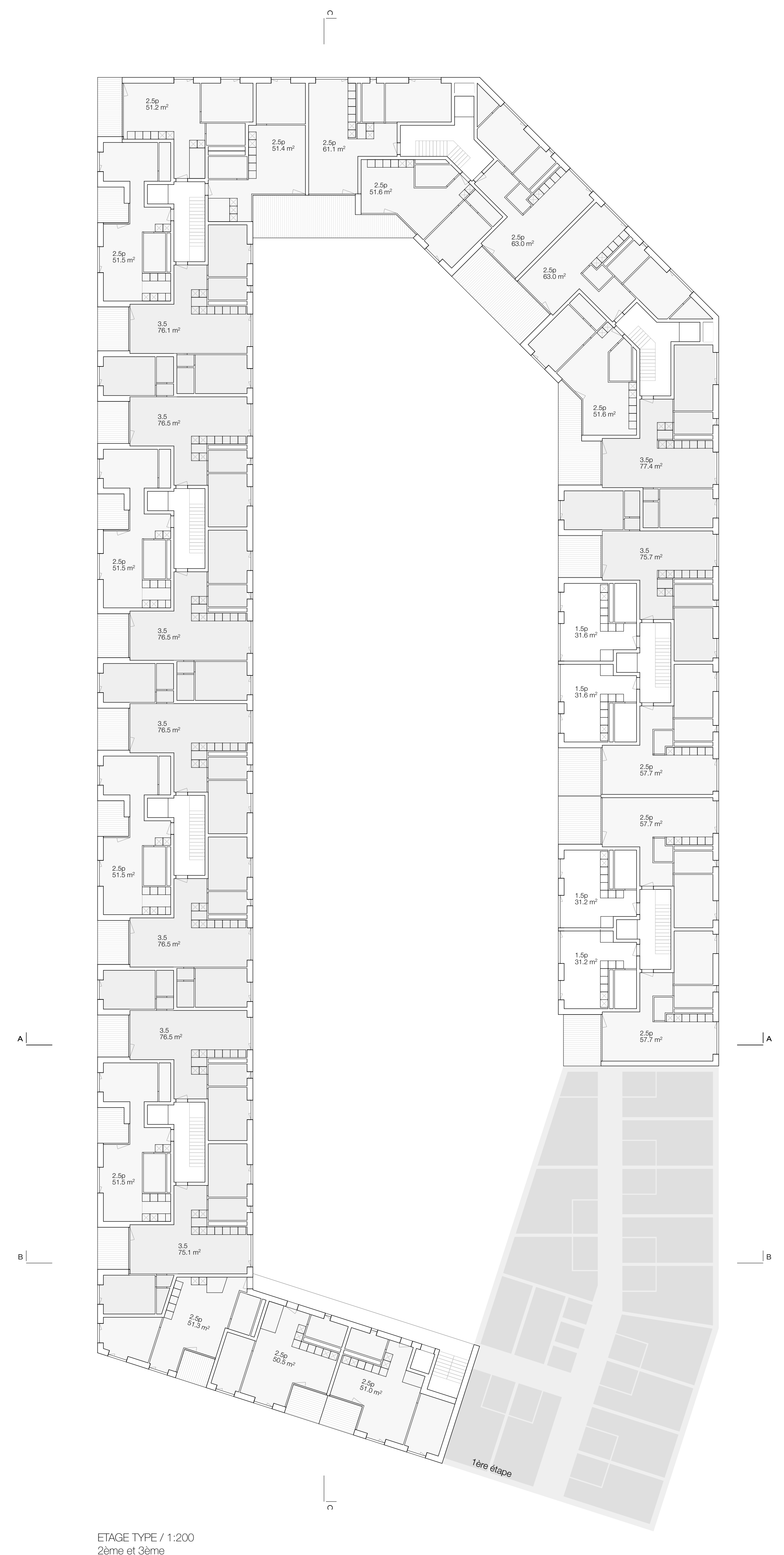
ETAGE TYPE / 1:200 2ème et 3ème
