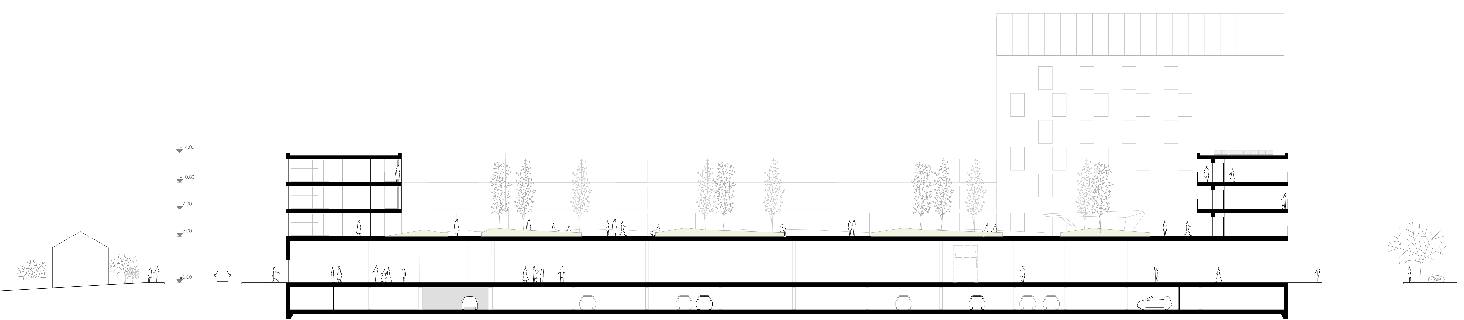
COUPE CC 1:200
