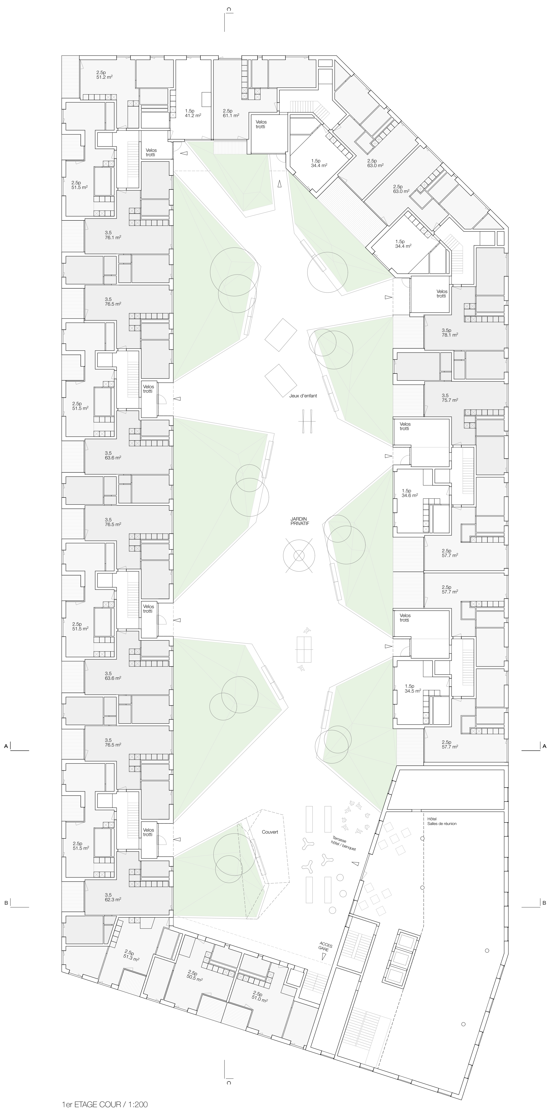
1er ETAGE COUR / 1:200
